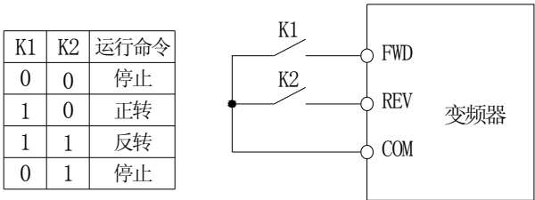
1. 二线制运转控制示意图
