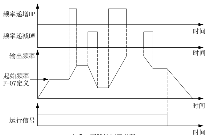
上升、下降控制示意图
